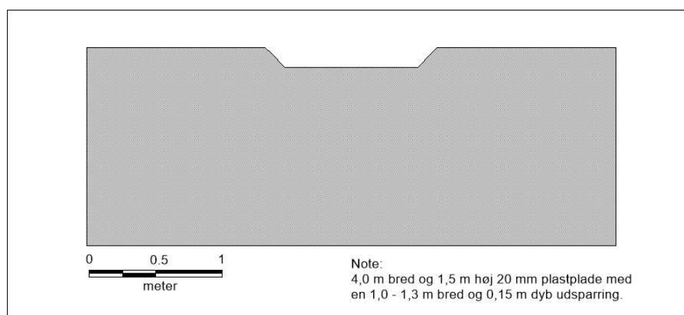
Figur 12. Skitse af en plastplade til brug som overløb i grøften i afløbet fra Sortemose og vist i skala 1:25.
