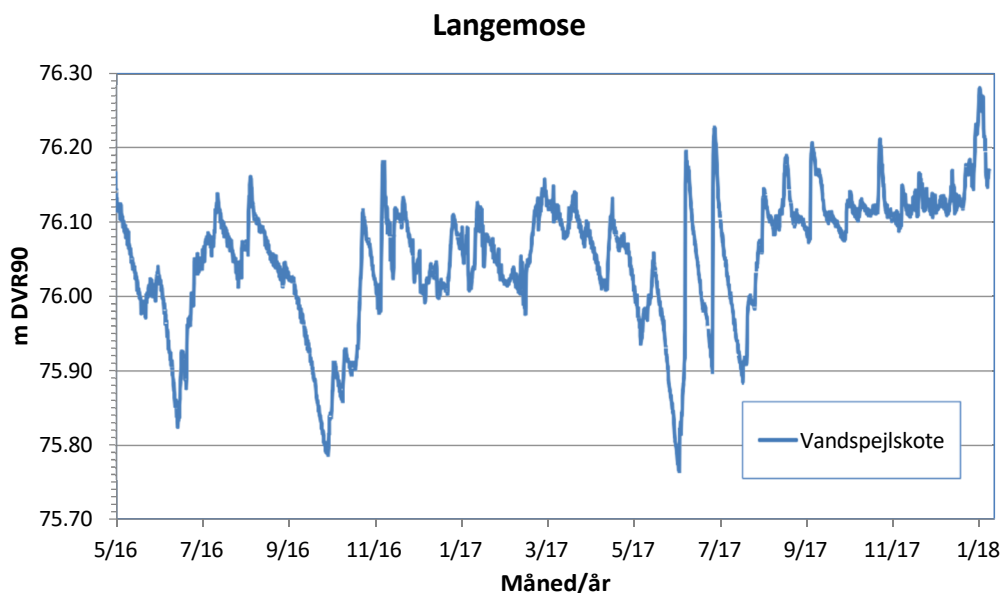
Figur 4. Kurve over det koterede vandspejlsforløb på den faste vandstandsmålestation i Langemose i perioden 1. maj 2016 til 11. januar 2018.
