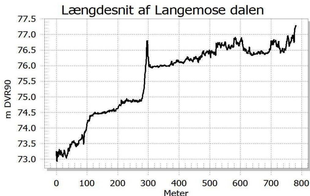
Figur 11. Terrænprofil fra den laserskannede højdemodel fra 2015 med et forløb på langs af dalen igennem Langemose fra den vestlige skovvej i afstand 0 til venstre og til højre mod øst til den østlige skovvej i afstanden 784 meter og udtrukket lidt syd for grøften igennem mosen.
