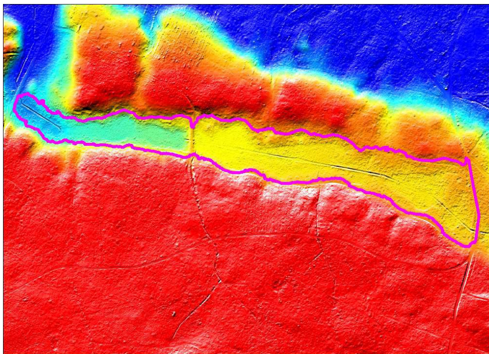
Figur 3. Den nye højdemodel af Langemose, som blev opmålt i 2015, vist i skala 1:6.000 med en højdebestemt farvelægning i en regnbueskala fra mørkeblå i kote 72,0 m, gul i kote 76,0 m og rød i kote 80,0 m og derved samt med en indlagt 30° belysning, der fremhæver terrænkonturerne. Man kan således se hver eneste grøft eller hjulspor i moseoverfladen med få centimeters nøjagtighed i en pixel-opløsning på kun 0,40 m, Styrelsen for Dataforsyning og Effektivisering ©. Kortet er vist i samme udsnit som på Figur 2 og med projektområdet i lys lilla omrids.
