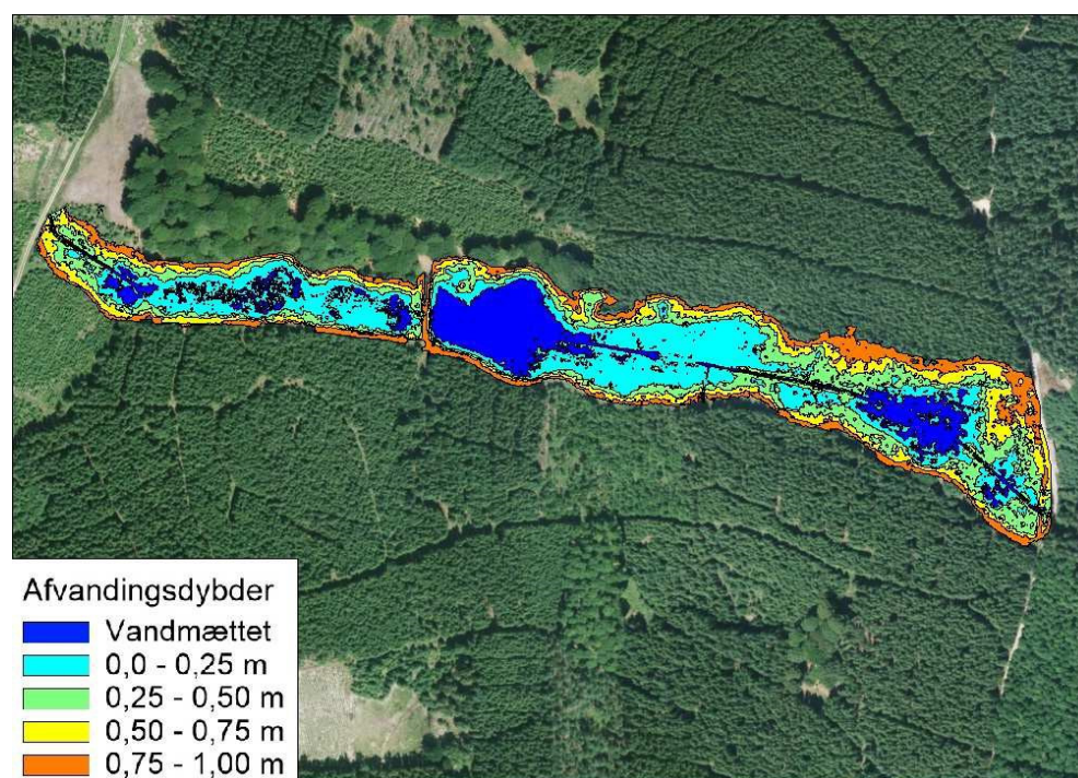
Figur 17. De beregnede afvandingsforhold i Langemose under de projekterede forhold med vandmættede arealer vist med mørkeblå farve og med 4 intervaller af afvandingsdybder per 0,25 m vist i skala 1:6.000 på baggrund af DDO®2016, ©COWI.
