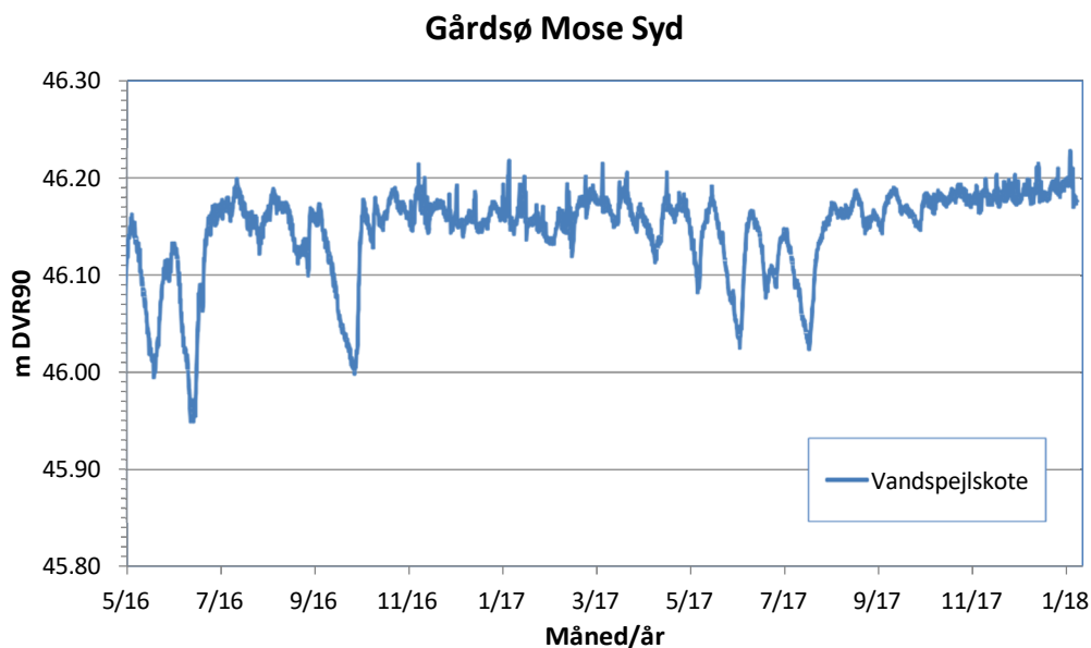
Figur 5. Kurve over det koterede vandspejlsforløb på den faste vandstandsmålestation i den sydlige del af Gårdsø Mose i perioden 1. maj 2016 til 11. januar 2018.
