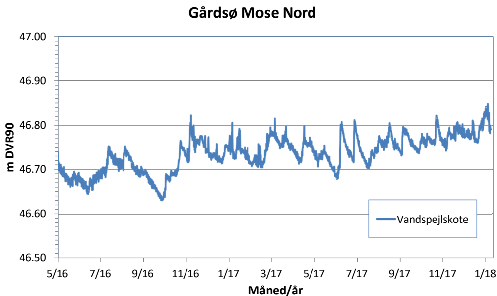
Figur 4. Kurve over det koterede vandspejlsforløb på den faste vandstandsmålestation i den nordlige del af Gårdsø Mose i perioden 1. maj 2016 til 11. januar 2018.
