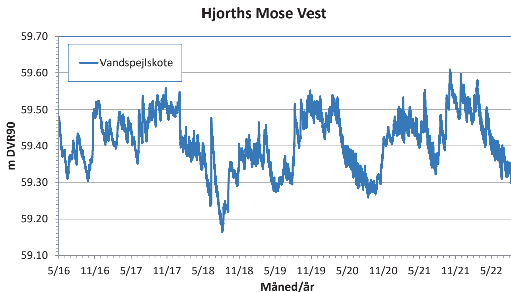
Figur 2. Kurve over det koterede vandspejlsforløb på vandstandsmålestationen i Hjorths Mose i perioden 1. maj 2016 til 24. august 2022.
