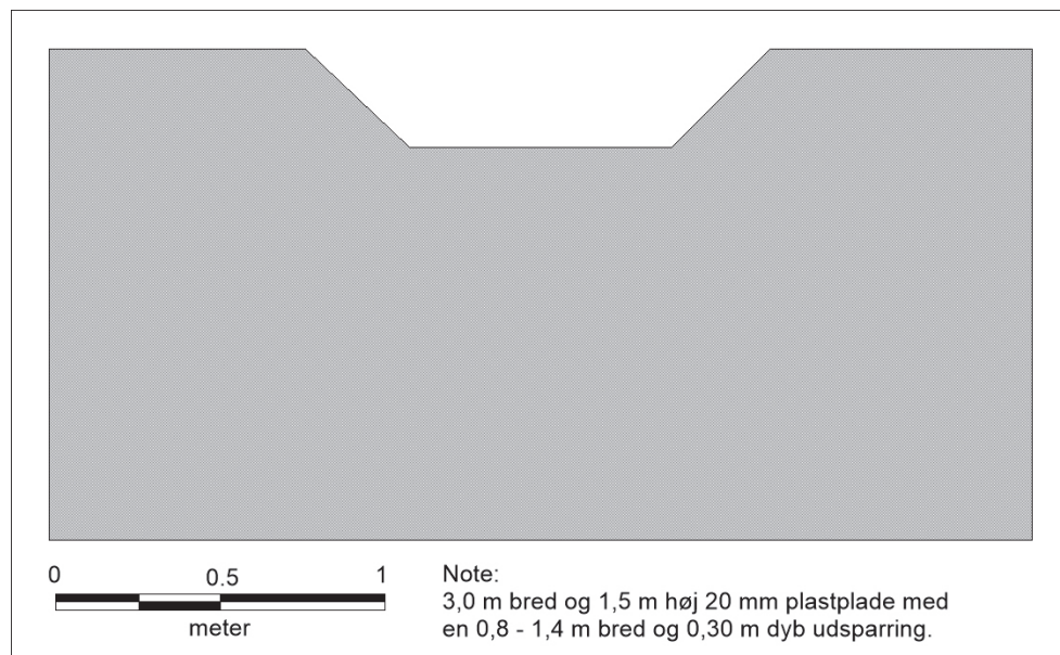
Figur 3. Skitse af en plastplade til brug som overløb i grøften fra den vestlige del af Hjorths Mose og vist i skala 1:25.
